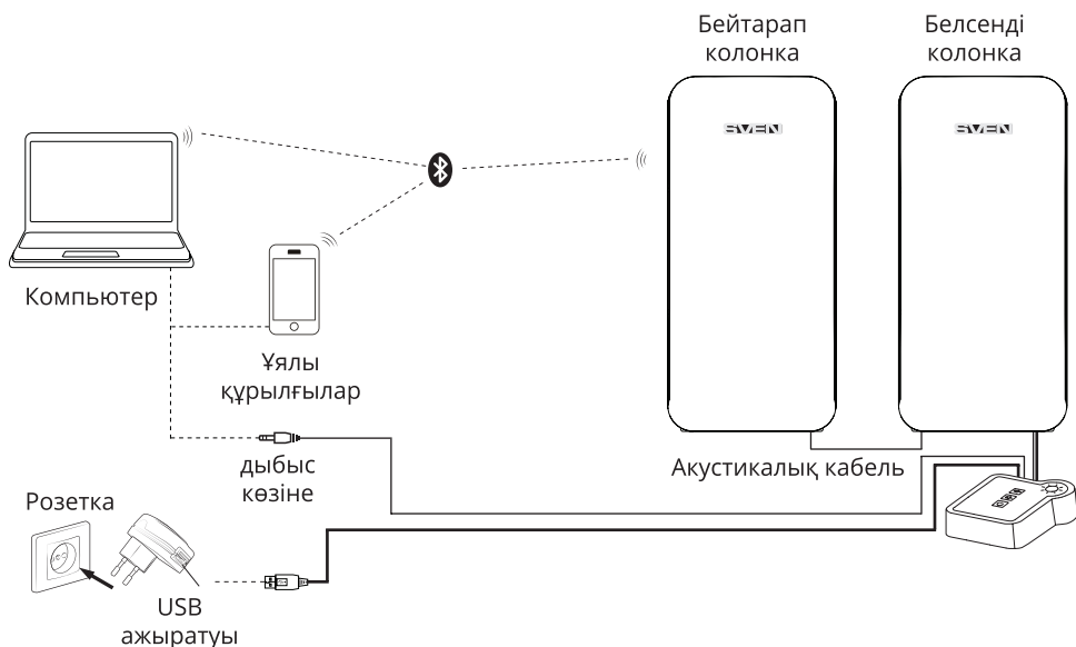
2-сурет. Қосылу схемасы
