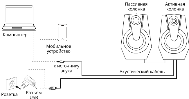
Рис. 2. Схема подключения
