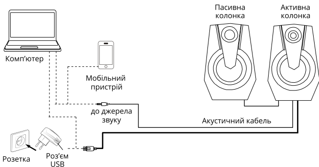
Мал. 2. Схема підключення
