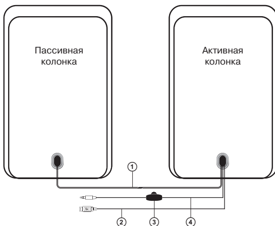
Рис. 1. Задние панели колонок
