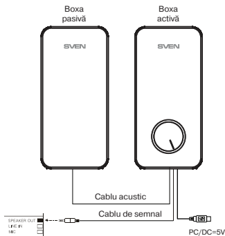
Imag. 2. Schema conectării
