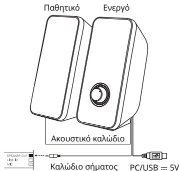
Εικ. 2. Σχέδιο σύνδεσης
