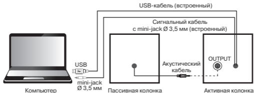
Рис. 2. Схема подключения
