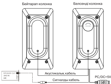
2-сурет. Қосу схемасы
