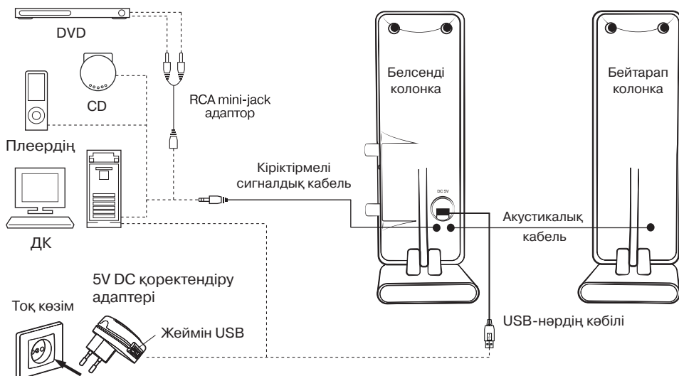
2-сурет. Қосылу схемасы
