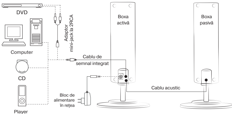
Imag. 2. Schema conectării
