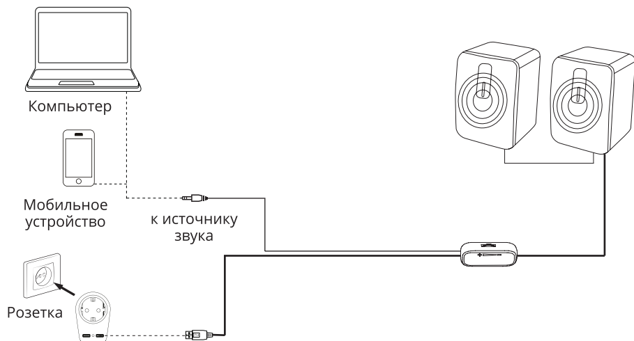
Рис. 2. Схема подключения
