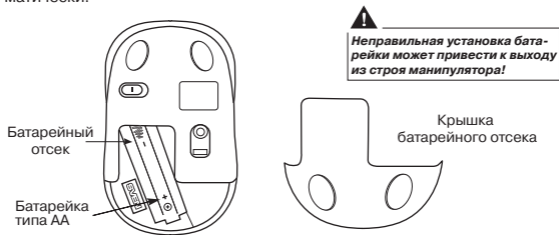
Рис. 4. Установка батарейки
