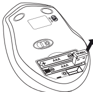
Imag. 7. Extragerea receiver-ului din carcasa mouse-ului
