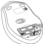
Imag. 6. Instalarea receiver-ului în carcasa mouse-ului
