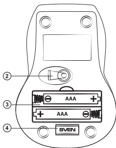
Рис. 2. Вид снизу
