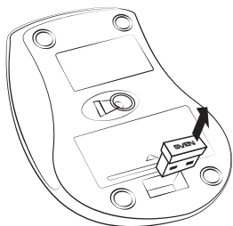
Мал. 5. Виймання ресивера з корпусу миші
