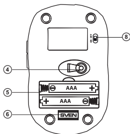
Рис. 2. Вид снизу
