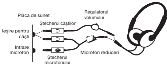
Imag. 1. Schema conectării
