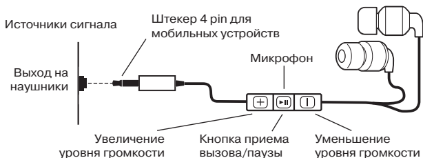
Рис. 1. Схема подключения
