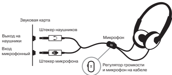
Рис. 1. Схема подключения
