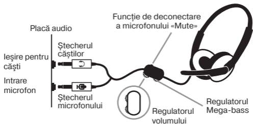
Imag. 1. Schema conectării
