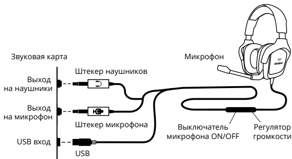
Рис. 1. Схема подключения
