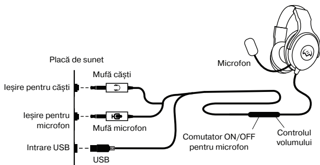
Fig. 1. Schema de conexiune
