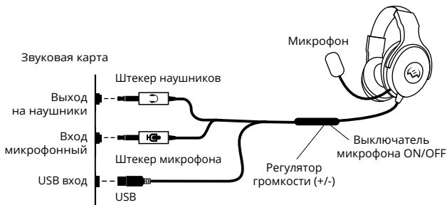
Рис. 1. Схема подключения
