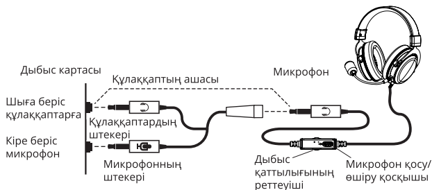
2-сурет. Қосылу схемасы
