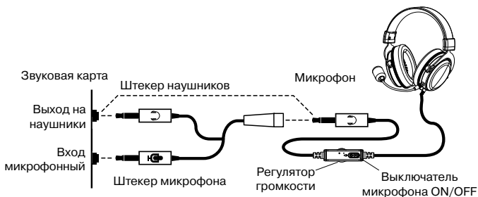
Рис. 2. Схема подключения
