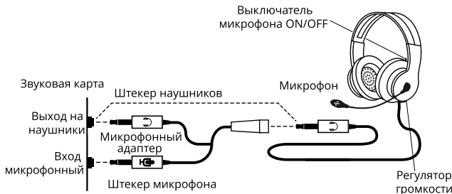
Рис. 1. Схема подключения
