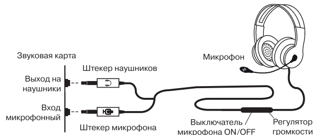
Рис. 1. Схема подключения
