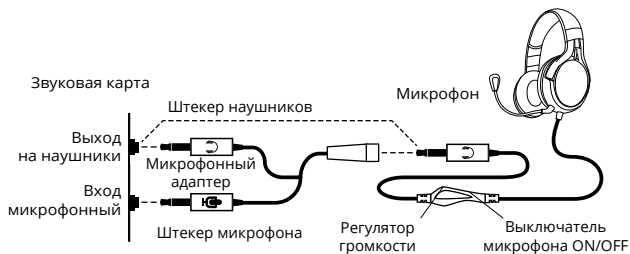
Рис. 2. Схема подключения
