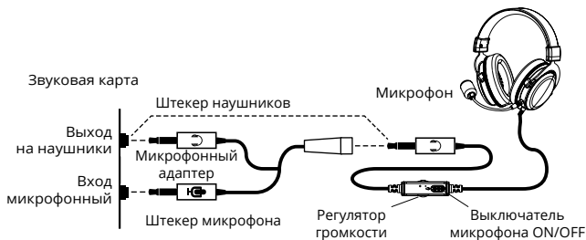
Рис. 2. Схема подключения
