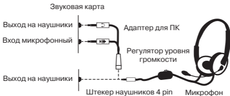
Рис. 1. Схема подключения
