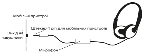
Мал. 1. Схема підключення
