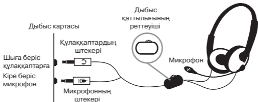
1-сурет. Қосылу схемасы
