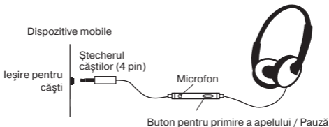
Imag. 1. Schema conectării
