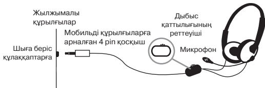
1-сурет. Қосылу схемасы
