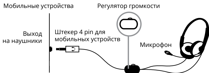
Рис. 1. Схема подключения
