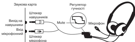
Мал. 1. Схема підключення
