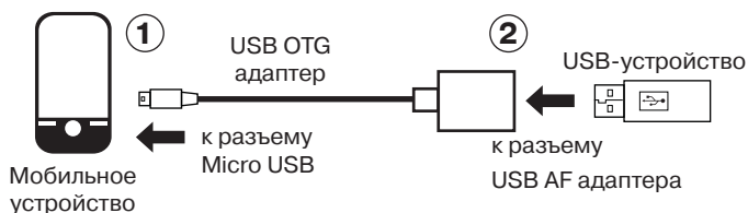
Схема подключения
