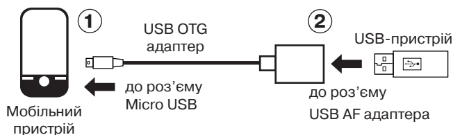
Схема підключення
