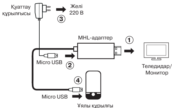
Қосылу схемасы
