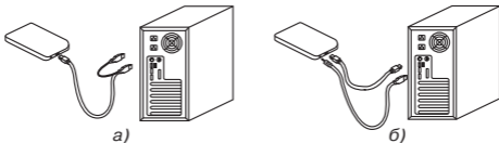
Мал. 2. Схеми підключення: а) по USB 2.0; б) по eSATA
