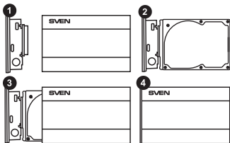
Мал. 1. Схема встановлення обладнання
