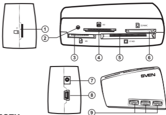
Мал. 1. Конструкція кардрідера (вигляд спереду, зверху, ззаду, збоку)
