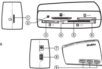
Рис. 1. Конструкция кардридера (вид спереди, сверху, сзади, сбоку)
