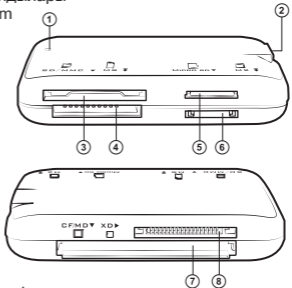
1-сурет. Кардридердің құрылысы
